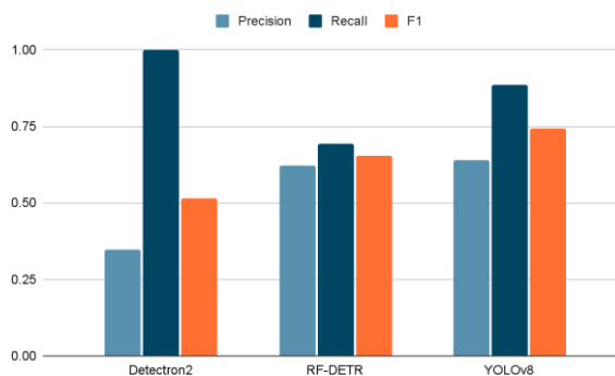
17-р зураг. Архитектурын харьцуулалтын график үр дүн
