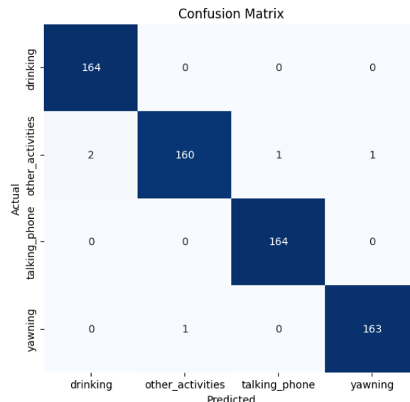
10 – р зураг. ViT архитектуртай загварын тестийн өгөгдөл дээрх гүйцэтгэл
