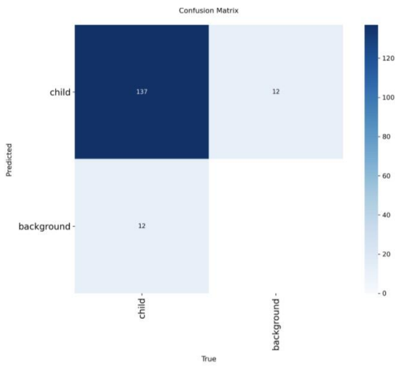
18-р зураг. YOLOv5 загварын төөрөгдлийн матриц
