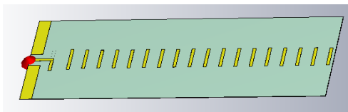
7-р зураг. Бичил туузан Яаги-Уда антенны 5.8 ГГц-ийн ажлын давтамж дээрх CST загварчлал
