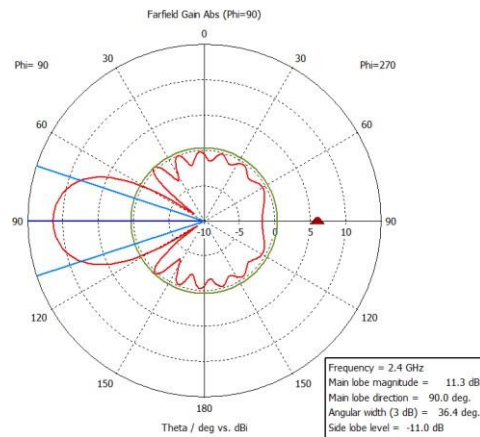
10-р зураг. 2.4 ГГц Антенны цацаргалтын диаграм
