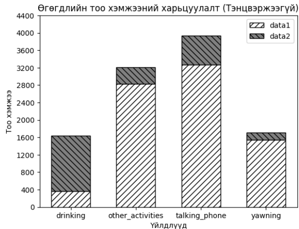
5 – р зураг. Тэнцвэргүй өгөгдлийн харьцуулалт
