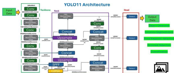
11-р зураг. YOLOv11 архитектур
