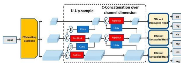
10-р зураг. YOLOv8 архитектур
