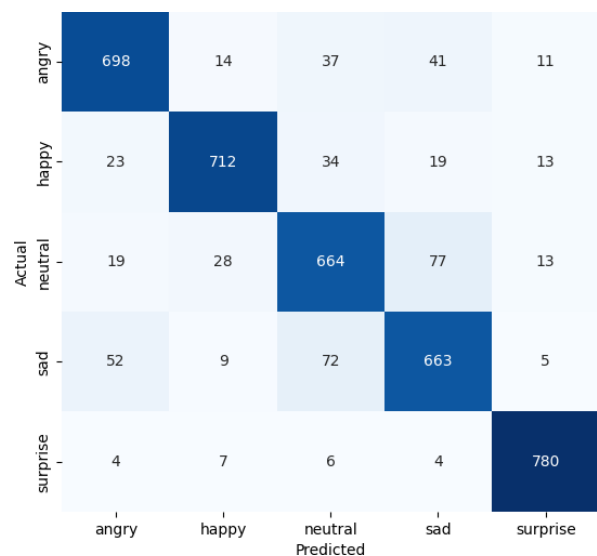
17 – р зураг. DeiT загварын тестийн багц дээрх төөрөгдлийн матриц
